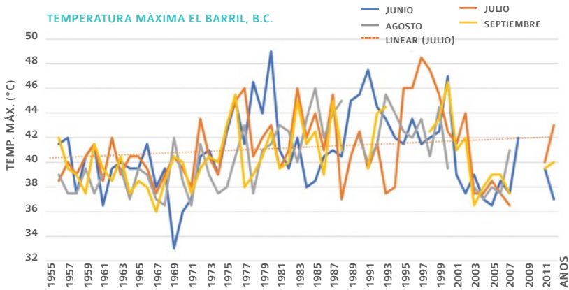
↑ Figura 14. Temperatura máxima registrada en la estación El Barril y línea de tendencia de julio.
