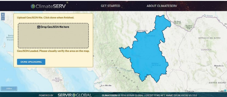
↑ Figura 3. Ingreso de archivo GeoJSON a la base de datos Climateserv para descarga de series de tiempo de precipitación (Servir Global, 2018).
