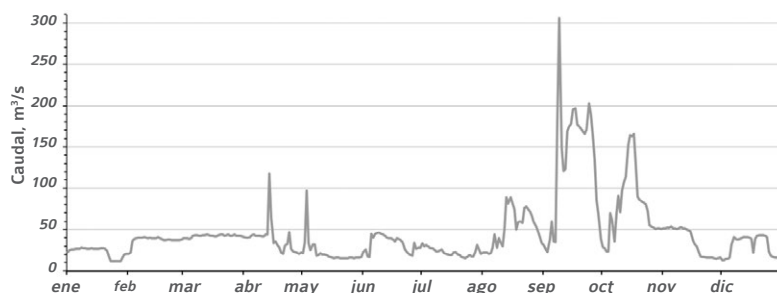
↑ Figura 6. Hidrograma del escurrimiento medio diario de la EH 24230-Ojinaga.
