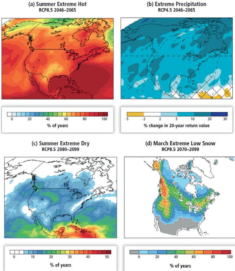
↑ Figura 4. a) Cambios en veranos extremadamente calientes, b) precipitaciones extremas, c) veranos extremadamente calientes, d) marcos con nieve extremadamente baja. Escenarios para dos horizontes de tiempo (mediados y finales de siglo) y para RCP8.5 (Romero-Lankao et al. , 2014).
