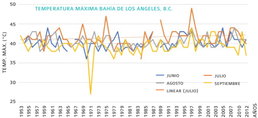
↑ Figura 10. Temperatura máxima registrada en la estación Bahía de los Ángeles y línea de tendencia de julio.
