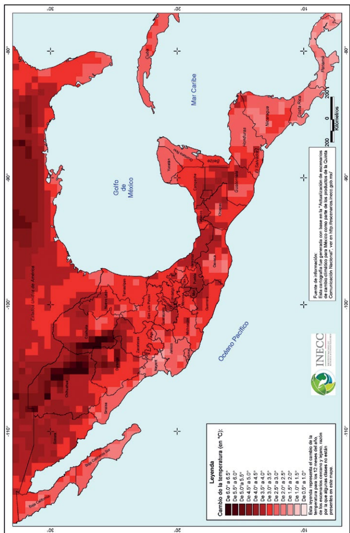
Figura 2. Anomalía de temperatura máxima para el mes de agosto, en el escenario RCP 6.0 (INECC, 2017).
