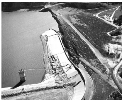
← Figura 4. Daños en la presa Lower Van Norman después del sismo de San Fernando (tomada de The San Fernando, California Earthquake of February 9, 1971 , por U. S. Geological Survey, 1971, United States Government Printing Office).
