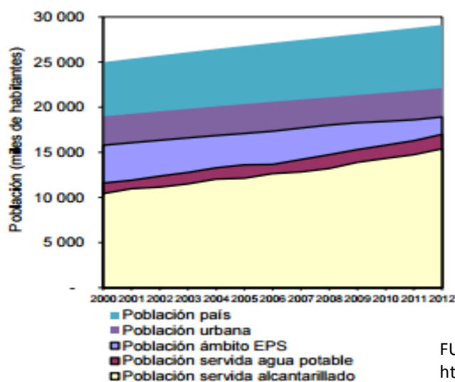
Gráfico N° 11: Cobertura de Agua Potable al 2013
